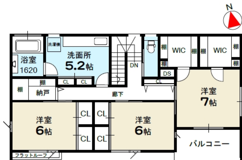
2階平面図
