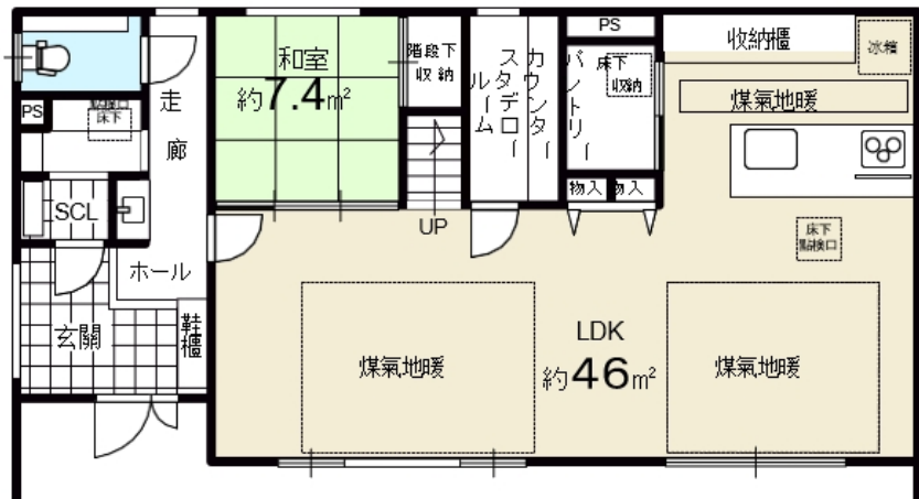
1層平面圖
